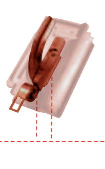
Hliníkové vodící a bezpečnostní střešní háky se zabudovaným tlumičem pádu, Typ A podle DIN EN 517
